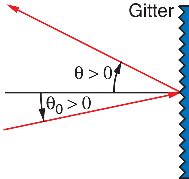
Vorzeichenkonvention am Reflexionsgitter
