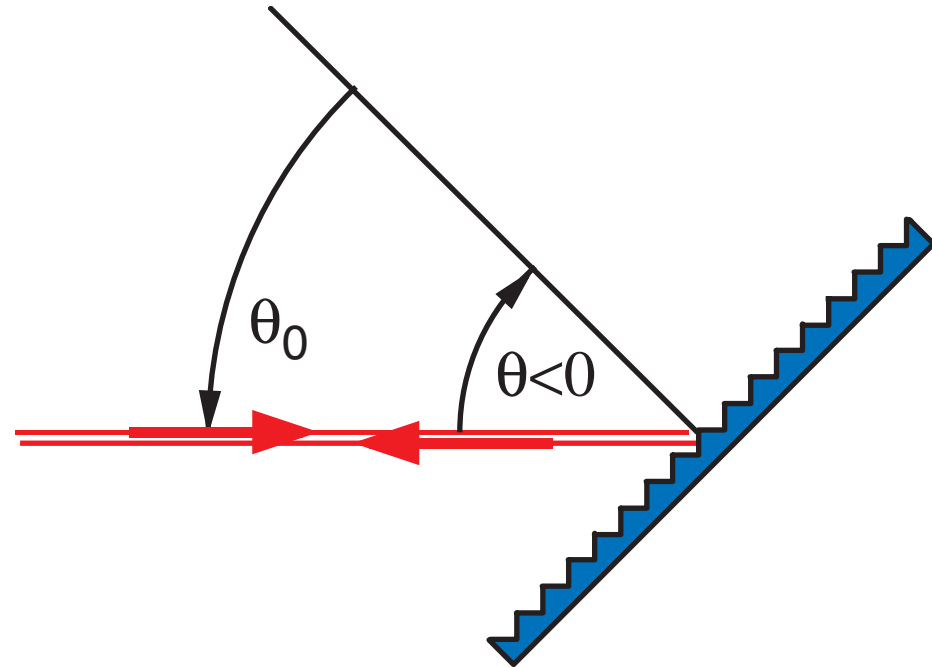
Littrow Anordnung \theta = -\theta_0
