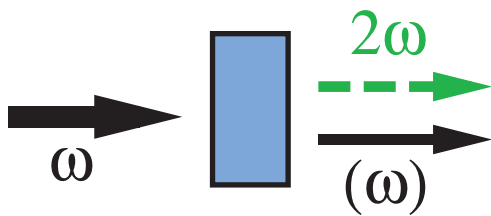
Frequenzverdopplung \omega + \omega = 2\omega
