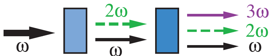
Technisch eingesetzte Frequenzverdreifachung \omega + \omega = 2\omega 2\omega + \omega = 3\omega
